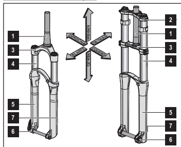
Figura 1 - Orientación convencional de la horquilla
