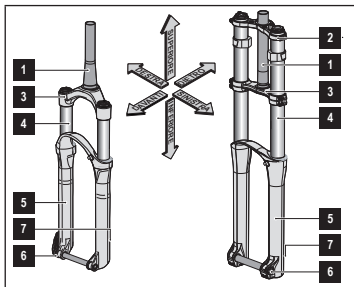
Figura 1 - Orientamento convenzionale della forcella
