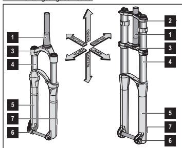
Abbildung 1 - Richtungsangaben Gabel
