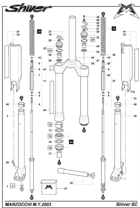
MARZOCCHI M.Y.2003 Shiver SC
