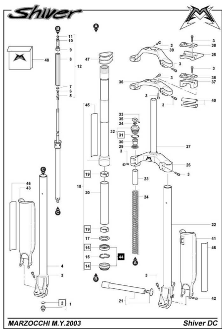
MARZOCCHI M.Y.2003 Shiver DC
