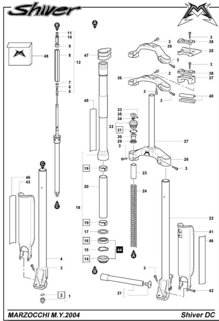
MARZOCCHI M.Y.2004 Shiver DC
