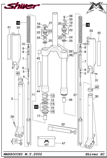
MARZOCCHI M.Y.2002 Shiver SC
