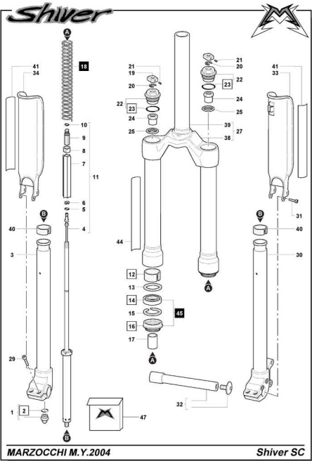
MARZOCCHI M.Y.2004 Shiver SC
