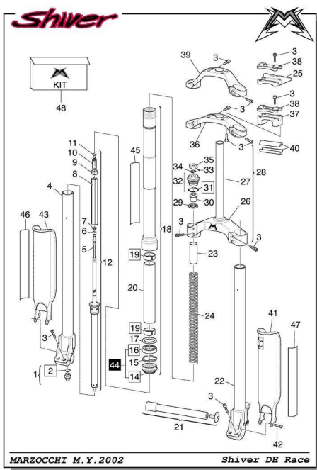
MARZOCCHI M.Y.2002 Shiver DH Race
