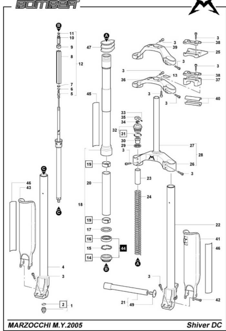
MARZOCCHI M.Y.2005 Shiver DC
