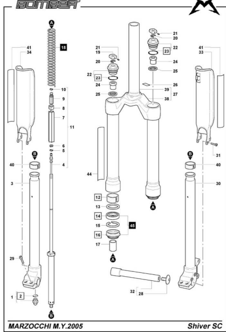
MARZOCCHI M.Y.2005 Shiver SC
