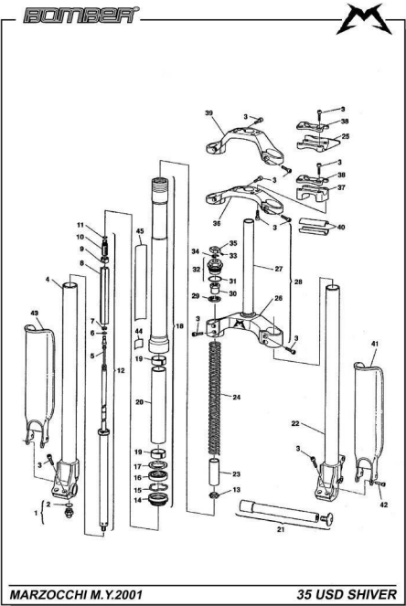
MARZOCCHI M.Y.2001 35 USD SHIVER
