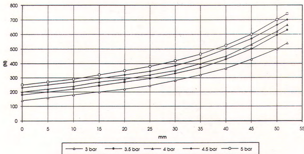
XC 500 carico statico della pressione
